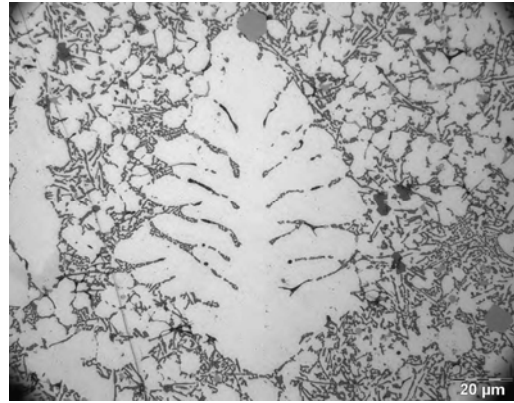
Weihnachtsbaum: Dendriten (Baum) und Schwerseigerungen (Kugel) in Aluminiumguss
